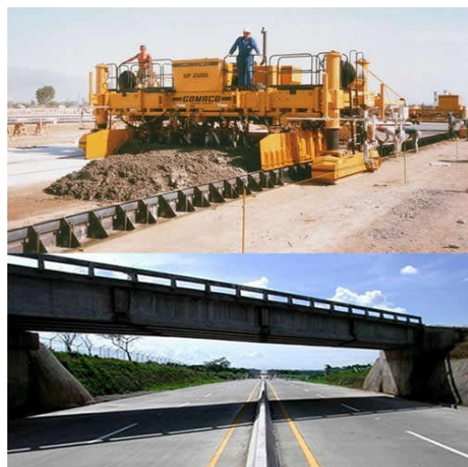
FIGURA 12-4: Pavimentadora
