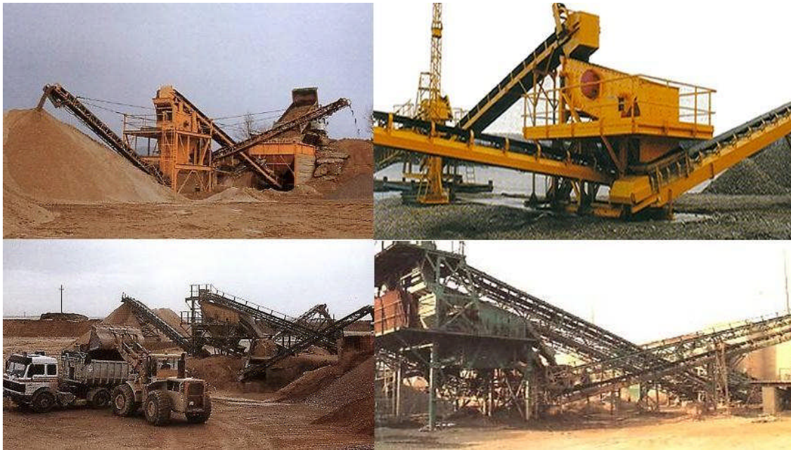
FIGURA 12-7: Planta de elaboracion de Aridos
