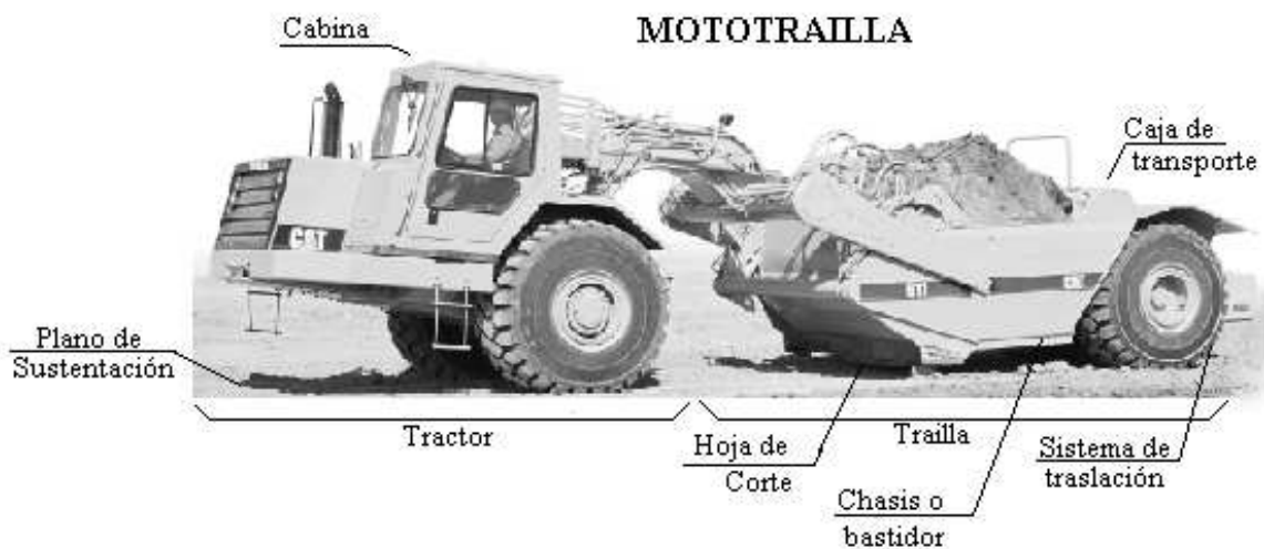
FIGURA 7-1: Partes Mototrailla
